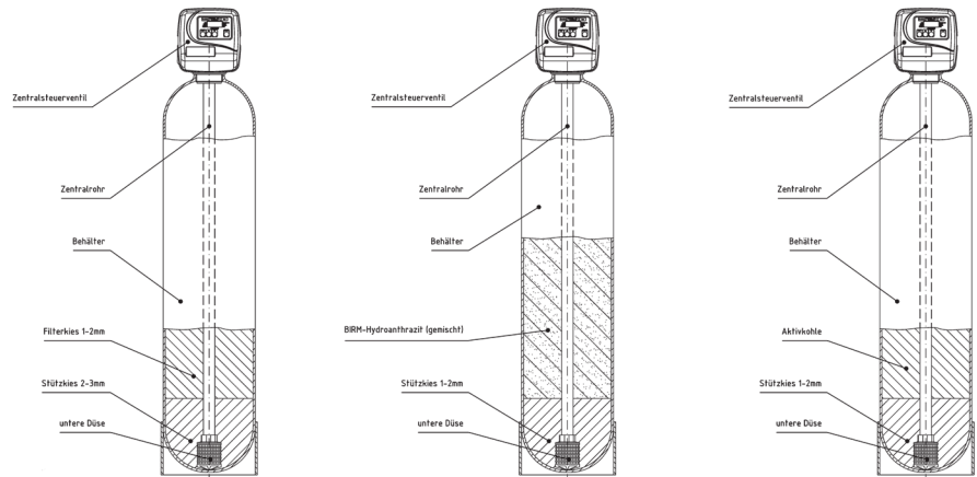
Grafik 1: Schnittzeichnung bei Patronenbehältern
